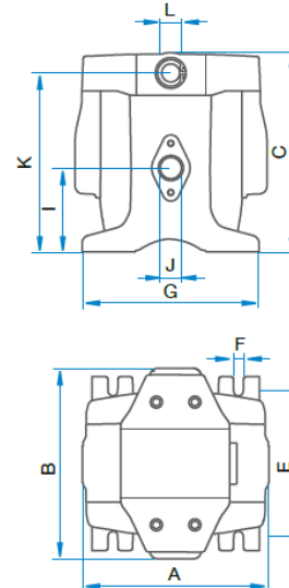
Abmessungen (mm)
